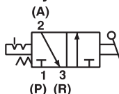
JIS Symbol
